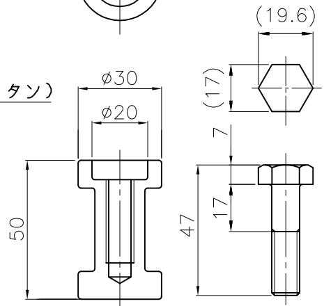
ボルト (M10X1.25P)
